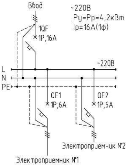
Рисунок 4.2 Схема линейная.
