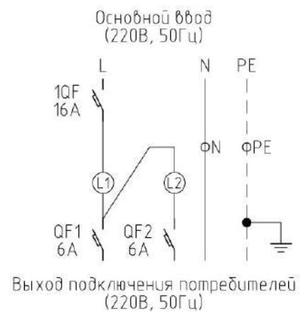
Рисунок 4.1 Схема подключения.
