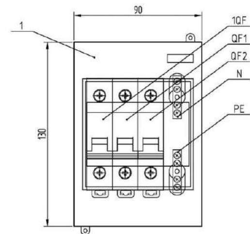
Рисунок 3.1 Компоновка изделия.
