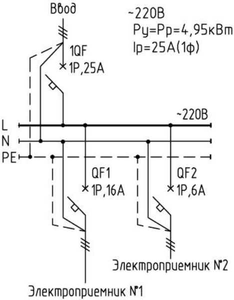
Рисунок 4.2 Схема линейная.
