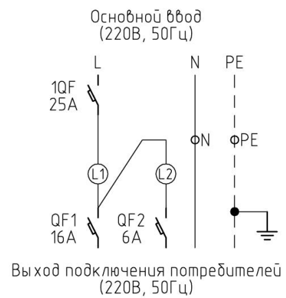
Рисунок 4.1 Схема подключения.
